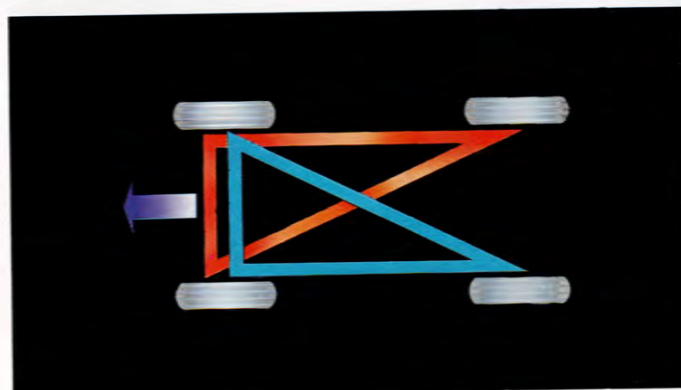
Volvo Taxi är utrustad med ett triangeldelat tvåkrets bromssystem. Bromsverkan med en krets är ca 80% av full effekt!
