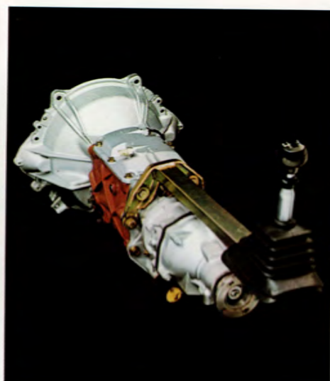
Växellådan är 4-växlad. GL-modellerna har dessutom överväxel som standard. Den ger lägre bränsleförbrukning och lägre ljudnivå. Automatlåda finns som alternativ.
