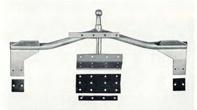
Draganordning 277979
