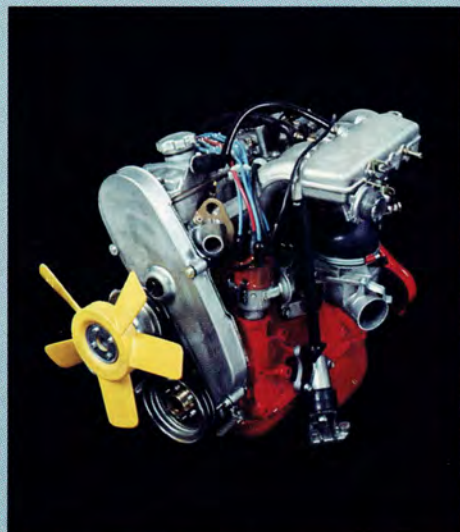
Accelerationssnabb motor, B 21 E, på 123 hk DIN vid 5.500 varv. Insprutning enligt CI-systemet. Brytarlöst elektroniskt tändsystem.
