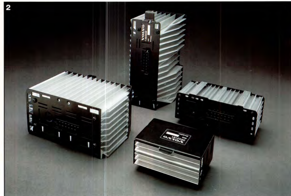
2. EFFEKTFÖRSTÄRKARE. I Volvo Sound System ingår ett brett sortiment av effektförstärkare, som ger möjligheter att bygga ett ljudsystem efter varje smak. Samtliga är utvecklade och byggda för Volvos bilar med tanke på att skapa både hög ljudkvalitet och snabb, säker montering. På bilden: HA-4240: 4x40W, HA-4140: 4x40W, HA-4120: 4x18W samt HA-2120: 2x20W.
