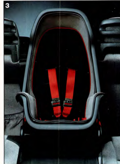
3. BARNSTOL FÖR BARN UPP TILL CA 4 ÅR. Stolen kan placeras på samtliga passagerar-platser i Volvo 960/940, 850, 740 och 240. På bilden är den mittplacerad bak. I övriga bilar – Volvo 460/440 och 480 – kan stolen placeras i passagerarsätet fram respektive på de två ytterplatserna bak.
