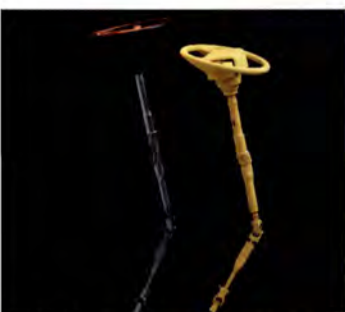
1975 – Kollapsfunktion, ratt/rattstång
