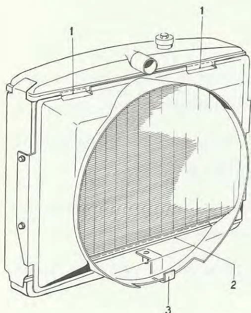
Bild 1. Flätkåpa monterad på kylare, vagn 140
