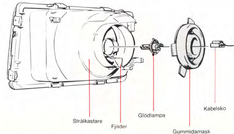
Gummidamask
