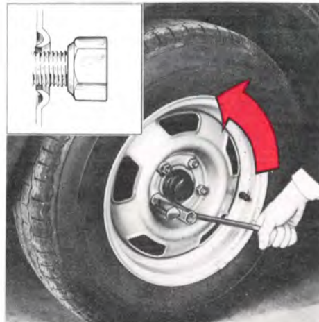
Lossa hjulmuttrarna
