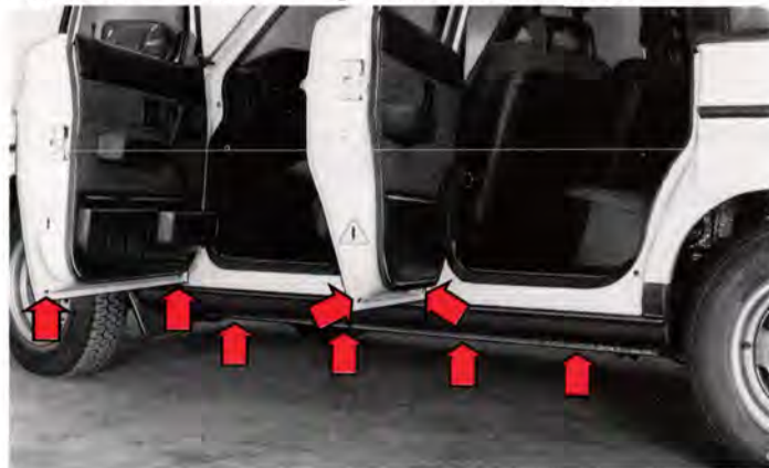
Dräneringshål
