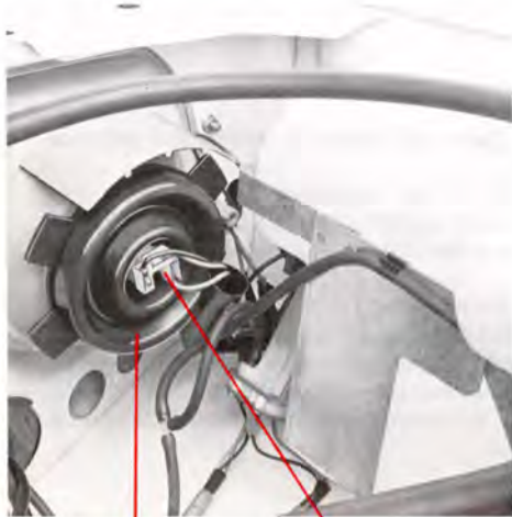
Gummidamask
