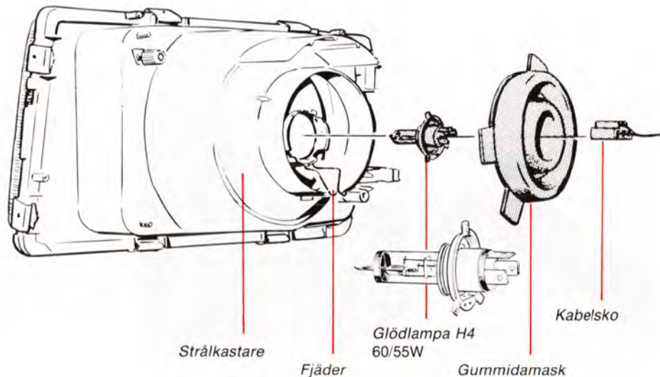
Fjäder
