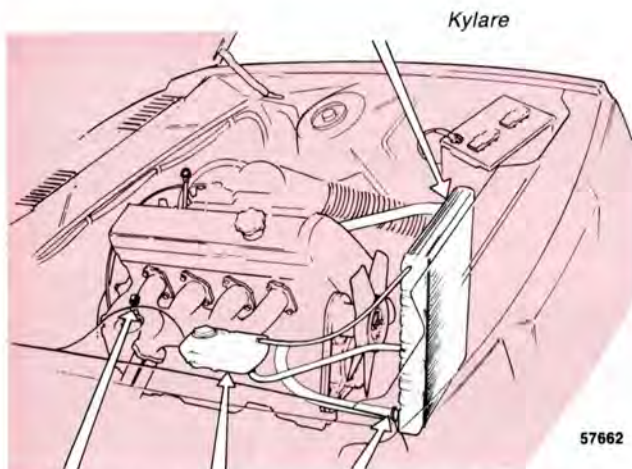
Avtappningskran Expansionstank Nedre kylarslang
