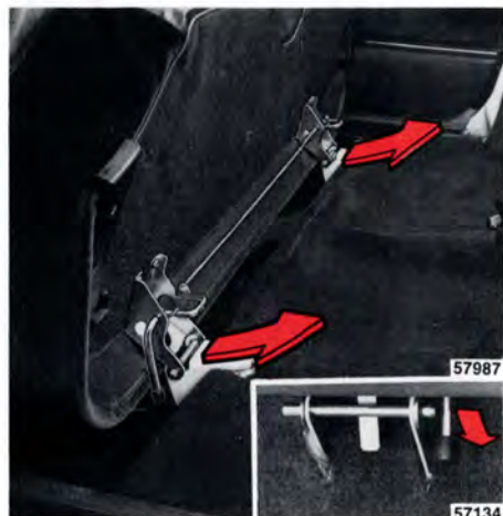
Ta bort sittedynan
