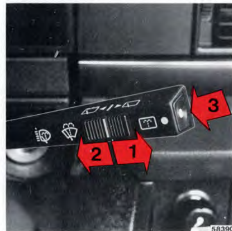
Reglage, bakrutetorkare
