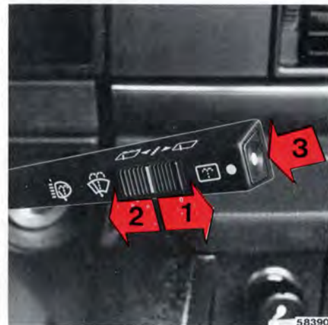
Reglage, bakrutetorkare
