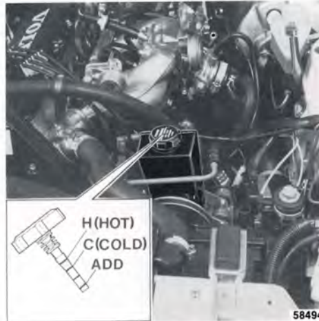
Oljemätsticka, servostyrning
